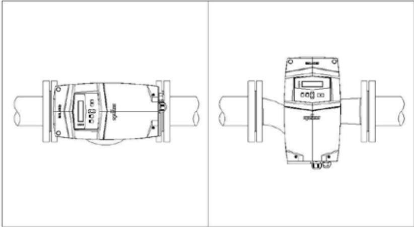
Şekil 6.3: Kontrol Kutusu Konum Değişikliği
