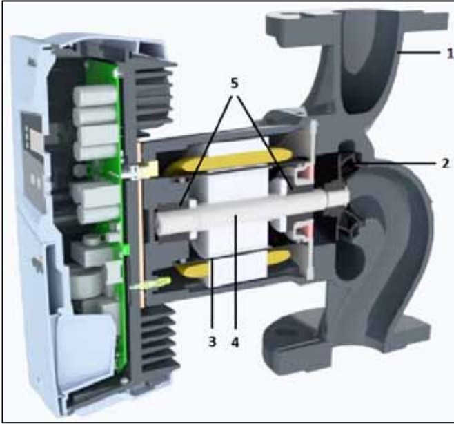
Şekil 3.1: Pompanın Kesit Resmi
